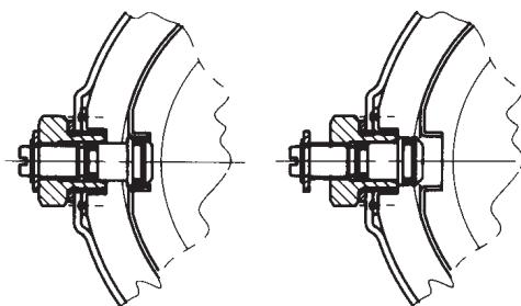
TAPÓN DE DRENAJE CON LA CLAVIJA CERRADA
