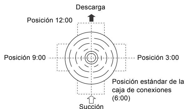
Fig. 11 Posiciones de la caja de conexiones del motor (vista superior)
