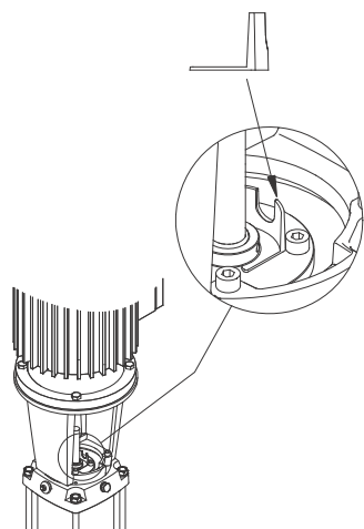
Fig. 19 Ajuste del acoplamiento para bombas CR y CRN 32, 45, 64, 90, 120 y 150
