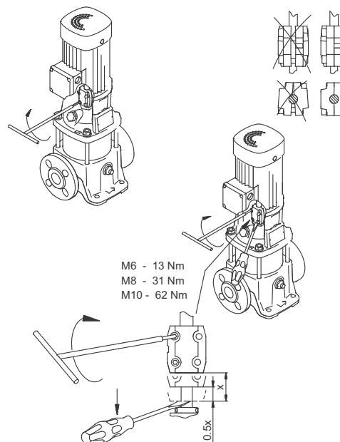
Fig. 17 Ajuste del acoplamiento para bombas CRT 2, 4, 8 y 16
