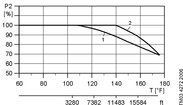
Fig. 3 Relación entre la potencia del motor (P2) y la temperatura ambiente/altitud
