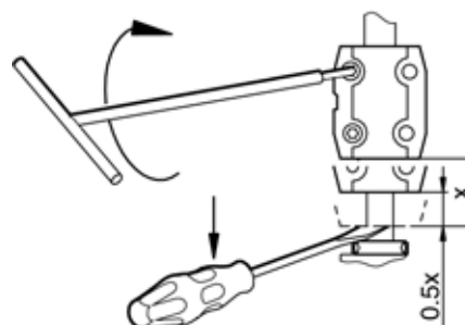
Fig. 18 Ajuste de las holguras del acoplamiento para bombas CRT 2, 4, 8 y 16
