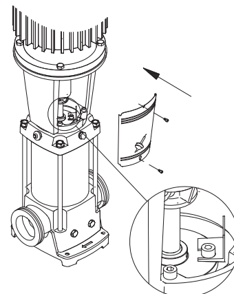
Fig. 21 Stockage de la fourche de réglage CR, CRN 32, 45, 64, 90, 120, et 150
