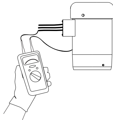
Fig. 26 Medida de la resistencia del aislamiento
